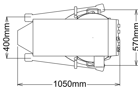
Boven aanzicht
