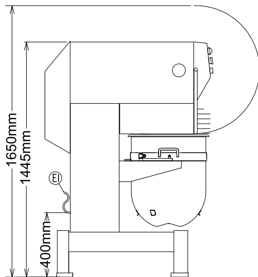
Zij aanzicht
